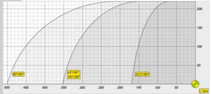
Diagrama de corte / Diagrama de corte Inclinación de las hojas, 90° / Inclinación das discos, 90°
