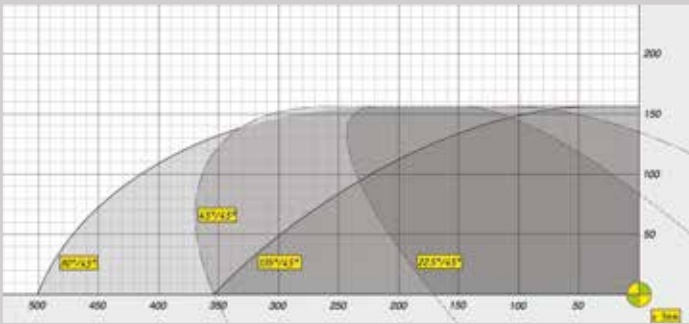
Diagrama de corte / Diagrama de corte Inclinación de las hojas, 45° / Inclinación das discos, 45°
