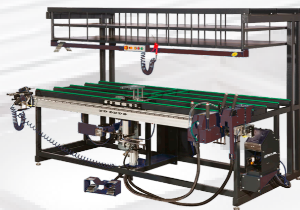
Banco de herrajes completo WS 131
