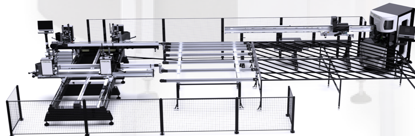
Línea automática de soldadura + enfriamiento + limpieza TURBO WELD 400
